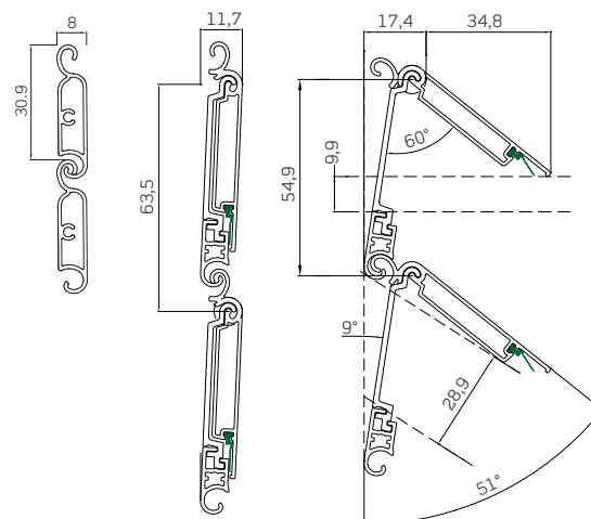
Sezione verticale
